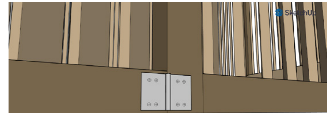
door detail: lower hinge
