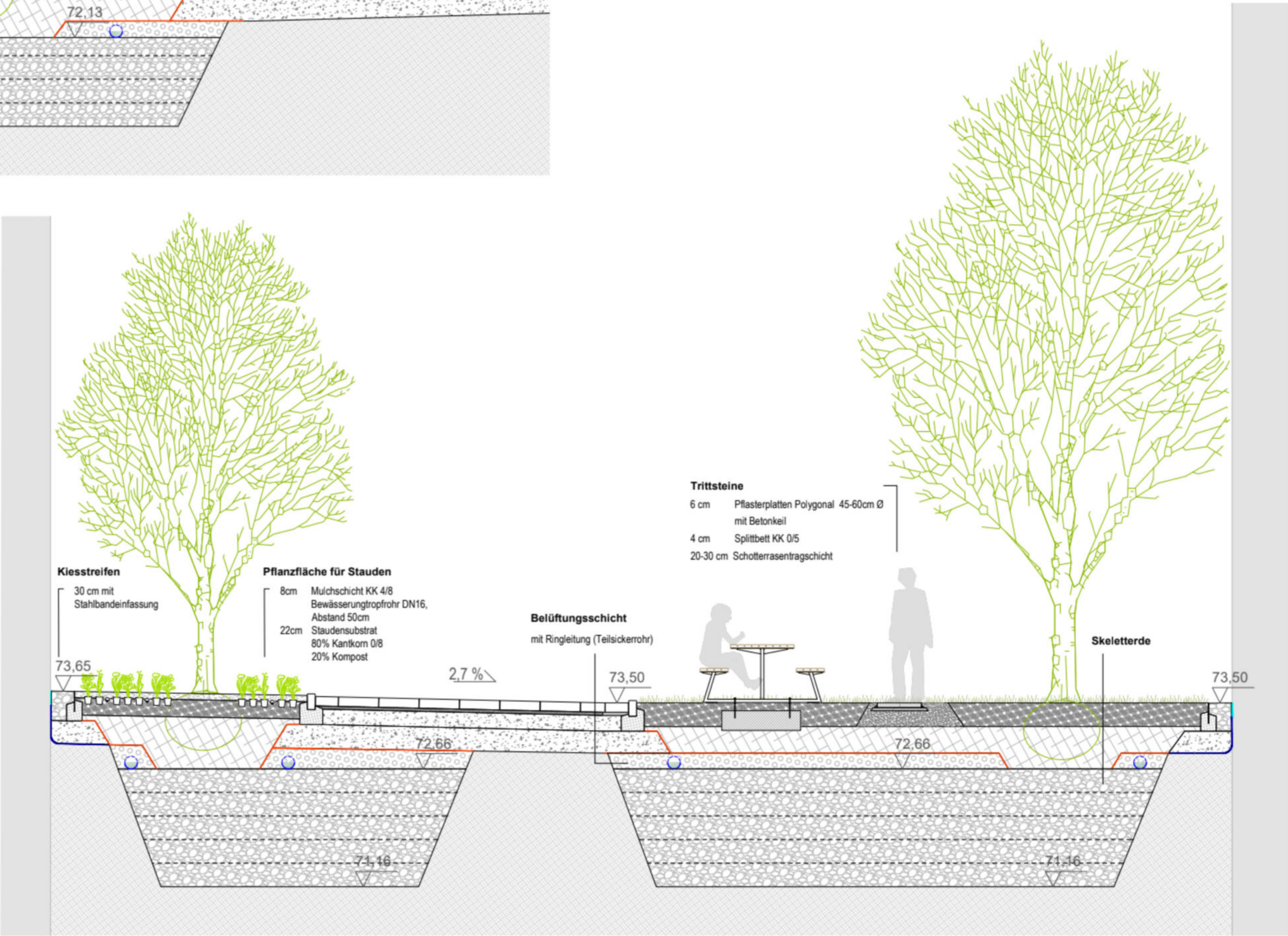
SCHNITT D 1:50
