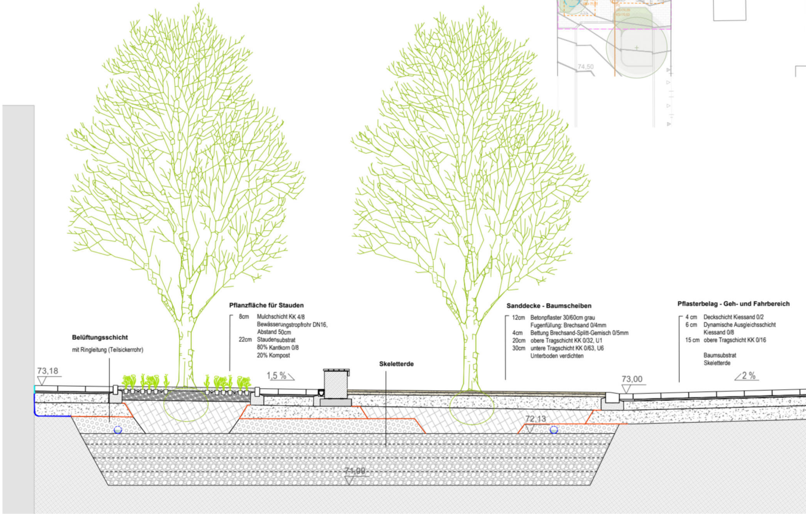
SCHNITT C 1:50
