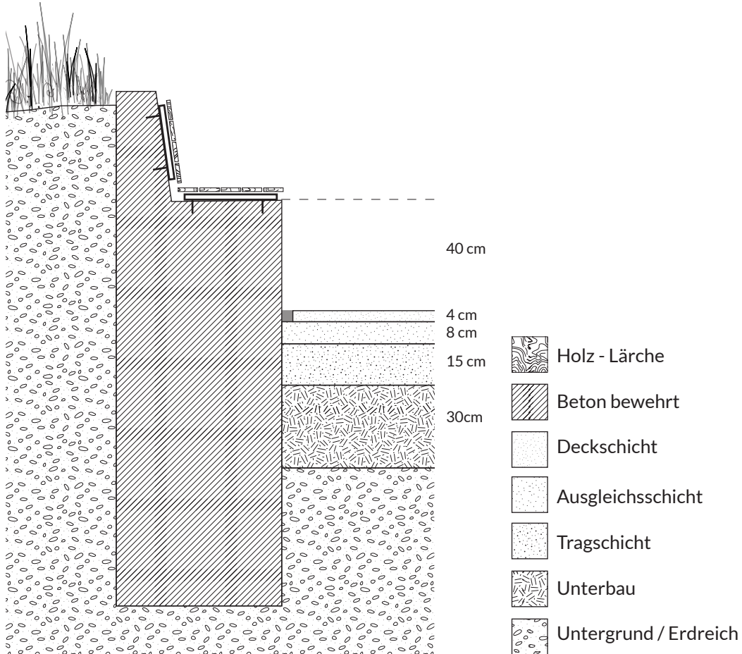
Detail Sitzbank / Stützmauer / Wassergebunde Decke M 1:20
